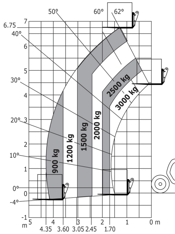
Lastdiagramm „Gelände“ (EN 1459 B)
